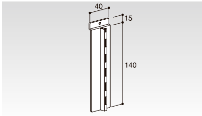
ブラケット用サポート(H140) (P-特長) HP-BKS40×140-Cr Cr:クロームメッキ W:ホワイト コードNo. 定価 色 55177 ¥1,880 Cr 梱50 160g 55197 ¥2,170 W
