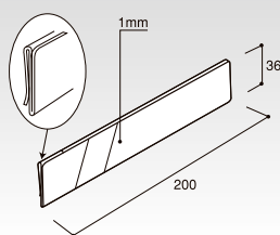
シューズフック用PCレール 透明塩ビ FU-PCR コードNo. 定 価 30g 55175 ¥770 ※FU型シューズフック専用
