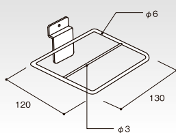
(P-U新) クロームメッキ シューズフック HP-SSHK コードNo. 定 価 重(g) 55138 ¥1,570 185g 棚30
