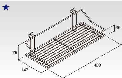
ミニバスケット (P-長) クロームメッキ HP-MBSK-N コードNo. 定 価 800g 55151 ¥7,500
