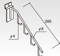
(P-中) クロームメッキ 袋物フック HP-FHK コードNo. 定 価 重(g) 242g 55132 ¥2,730 棚30
