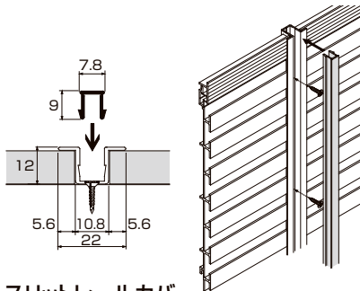
スリットレールカバー HL-SRC 2730 W
