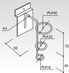
(P-大) クロームメッキ リングフック 3連 HP-R3HK コードNo. 定 価 重(g) 145g 55102 ¥3,500 棚30
