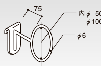
(P-大) クロームメッキ 垂直リングフック HL-V50RHK 内径(mm) コードNo. 定 価 重(g) 50 62083 ¥2,100 106 100 62084 ¥2,450 140 (棚30)
