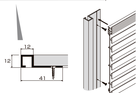
90°コーナレール
