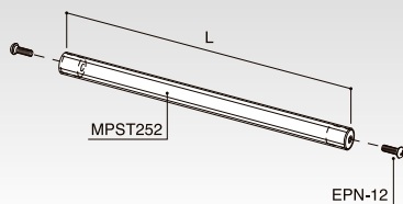
丸パイプセット クロームメッキ HP-MPST-585 L(mm) コードNo. 定 価 重さ(g) 585 55171 ¥1,560 392 885 55173 ¥1,810 590
