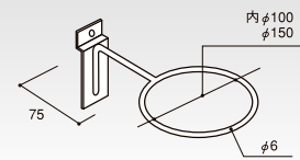
(P-小) クロームメッキ リングフック HP-100 RHK 内φ(mm) コードNo. 定 価 重(g) 100 55111 ¥2,520 137 150 55112 ¥2,730 173 棚50
