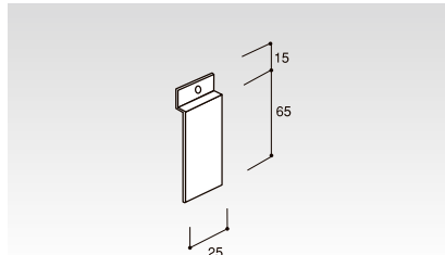
プレート生地(W25×H65) (P-小) HP-PT25×65N コードNo. 定価 梱100 36g 55180 ¥280
