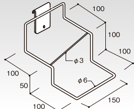
(P-U新) クロームメッキ シューズフック(2段/左傾斜) HL-SWHK/L コードNo. 定 価 重(g) 265g 62112 ¥2,220 (棚15)
