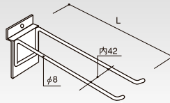
(P-大) クロームメッキ ダブルフック HP-WHK-200 コードNo. 定 価 重(g) 200 55091 ¥1,770 274 250 55092 ¥2,100 313 300 55093 ¥2,440 354 棚30
