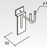
(P-小) クロームメッキ ネクタイフック HP-NTHK コードNo. 定 価 重(g) 51g 55101 ¥1,120 棚50
