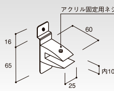
アクリル棚用ブラケット (P-専) クロームメッキ HP-ACBK コードNo. 定 価 100g 55174 ¥3,280
