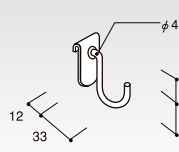
U型フック (P-小) HL-UHK クロームメッキ (棚100) 26g 62025 ¥1,050
