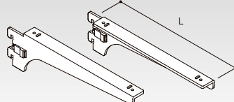
木棚ブラケット一体型(SP) (右・左セット) クロームメッキ NX443/L-R-120 SP L(mm) コードNo. 定 価 重さ(g) 120 76939 ¥1,050 280 170 76940 ¥1,170 320 220 76941 ¥1,300 390 ※ブラケット用サポートが必要です。
