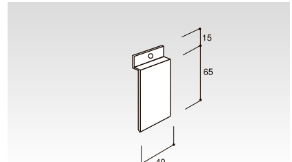
プレート生地(W40×H65) (P-中) HP-PT40×65N コードNo. 定価 梱100 60g 55179 ¥310
