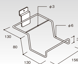
(P-U新) クロームメッキ FU型シューズフック(2段) HP-SWHK-FU コードNo. 定 価 重(g) 55136 ¥2,030 300g 棚15
