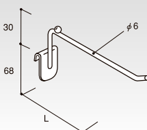
アップフック (P-大) HL-UPHK-150 クロームメッキ (棚50) L(mm) コードNo. 定 価 重さ(g) 150 62045 ¥840 94 200 62046 ¥960 107 250 62047 ¥1,100 117
