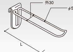
ダブルハンガー 巾30 (P-大) HL-WHG30-150 クロームメッキ (棚30) L(mm) コードNo. 定 価 重さ(g) 150 62051 ¥1,330 100 200 62052 ¥1,380 115 250 62053 ¥1,660 130
