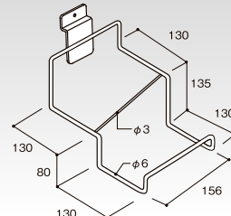
(P-U新) クロームメッキ FU型シューズフック(2段/左傾斜) HP-SWHK/L-FU コードNo. 定 価 重(g) 55137 ¥2,130 330g 棚15
