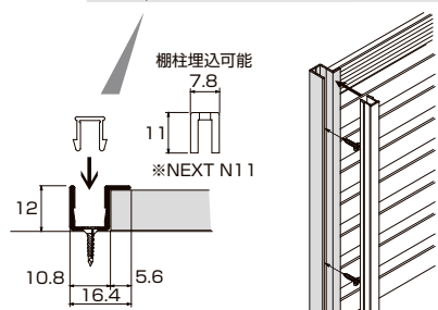
サイドスリットレール
