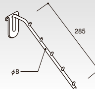
(P-大) クロームメッキ 傾斜フック HL-KSHK コードNo. 定 価 重(g) 195g 62091 ¥2,290 (棚30)
