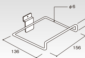
(P-U新) クロームメッキ FU型シューズフック HP-SSHK-FU コードNo. 定 価 重(g) 55135 ¥1,960 197g 棚30
