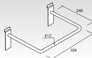
ホール用フック (P-特長) クロームメッキ HP-WLHK コードNo. 定 価 895g 55152 ¥6,160
