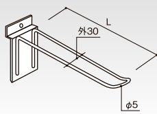
(P-中) クロームメッキ ダブルハンガー 巾30 HP-WHG30-150 コードNo. 定 価 重(g) 150 55086 ¥1,250 125 200 55087 ¥1,320 141 250 55088 ¥1,680 156 棚30
