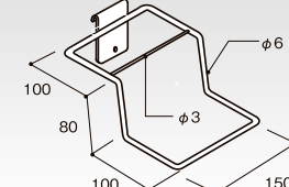
(P-U新) クロームメッキ シューズフック(2段) HL-SWHK コードNo. 定 価 重(g) 255g 62111 ¥1,890 (棚15)
