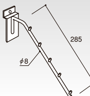
(P-中) クロームメッキ 傾斜フック HP-KSHK コードNo. 定 価 重(g) 210g 55131 ¥2,640 棚30
