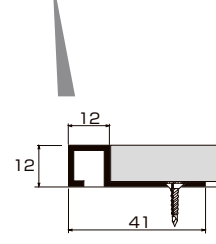
90°コーナレール HL-90CR 2730 W
