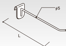
シングルフック φ5 (P-小) HL-HK5-100 クロームメッキ (棚100) L(mm) コードNo. 定 価 重さ(g) 100 62021 ¥470 37 150 62022 ¥520 46 200 62023 ¥560 51 250 62024 ¥620 59
