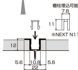
センタースリットレール HL-CSR 2730 W
