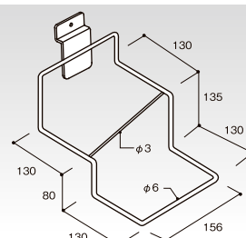
(P-U新) クロームメッキ シューズフック(2段/左傾斜) HP-SWHK/L コードNo. 定 価 重(g) 55140 ¥2,090 320g 棚15
