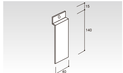
プレート生地(H140) (P-特長) HP-PT40×140N コードNo. 定価 梱100 115g 55181 ¥470
