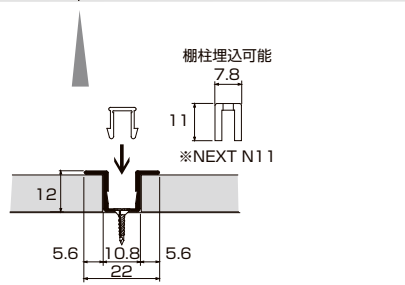
センタースリットレール
