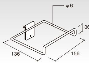
(P-U新) クロームメッキ FU型シューズフック HL-SSHK-FU コードNo. 定 価 重(g) 205g 62115 ¥1,940 (棚15)
