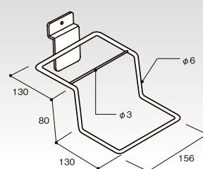
(P-U新) クロームメッキ シューズフック(2段) HP-SWHK コードNo. 定 価 重(g) 55139 ¥1,820 285g 棚15
