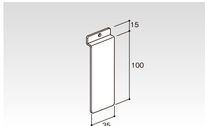
プレート生地(H100) (P-長) HP-PT35×100N コードNo. 定価 梱100 75g 55186 ¥420
