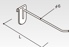
シングルフック φ6 (P-大) HL-HK6-150 クロームメッキ (棚50) L(mm) コードNo. 定 価 重さ(g) 150 62041 ¥590 84 200 62042 ¥620 95 250 62043 ¥680 107
