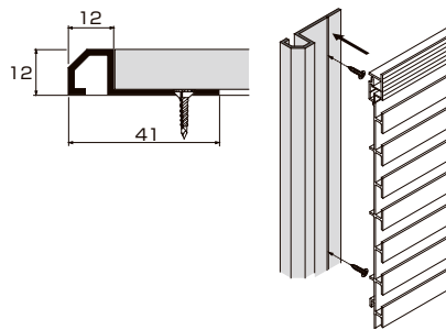
45°コーナレール
