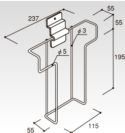
マガジンフック (P-U大) クロームメッキ HP-MZHK コードNo. 定 価 266g 55150 ¥3,220
