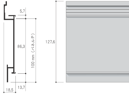
HP100S 1210 S 塩ビシートサイズ(目安) H89mm 0.90kg/m
