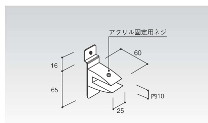
36 アクリル用ブラケット (P-専) クロームメッキ HP-ACBK コードNo. 定 価 100g 55174 ¥2,340 (棚50)
