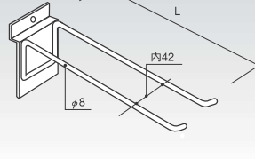
14 ダブルフック (P-大) クロームメッキ L(mm) コードNo. 定価 重量(g) 200 55091 ¥1,260 274 250 55092 ¥1,500 313 300 55093 ¥1,740 354 HP-WHK-200 (棚30)
