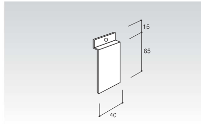
41 プレート 生地
