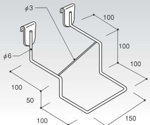
25 シューズフック (P-大) クロームメッキ コードNo. 定価 62112 ¥1,580 HL-SWHK/L (左傾斜) 265g (棚15)
