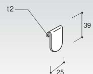
36 プレート 生地
