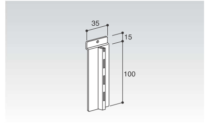
46 ブラケット用サポート
