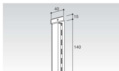
39 ブラケット用サポート (P-特長) Cr:クロームメッキ W:ホワイト HP-BKS40x140 コードNo. 定 価 色 55177 ¥1,340 Cr 55197 ¥1,550 W (棚50)
